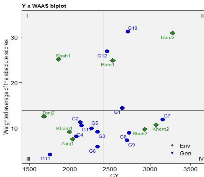
شکل ۳- بای پلات عملکرد دانه در مقابل میانگین وزنی نمرات مطلق برای بیشترین پیش‌بینی‌های ناریب خطی از اثر متقابل ژنوتیپ‌ها با محیط (WAASB)
